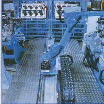
Asse movimentazione robot antropomorfo Antropomorphic robot linear unit
