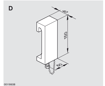
Piastra d'agganciamento
