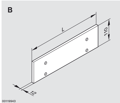
Piastra di attacco
