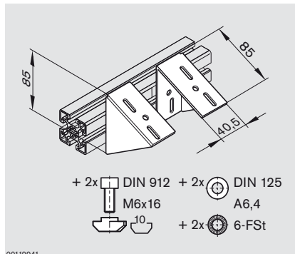
Angolare per fissare l'apparecchio di comando
