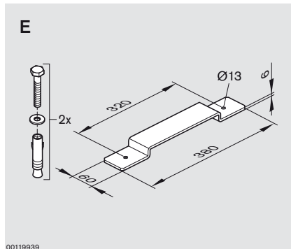
Piastrina d'appoggio
